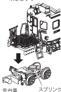
先台車
