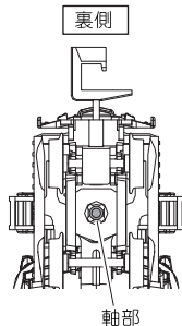
軸部
